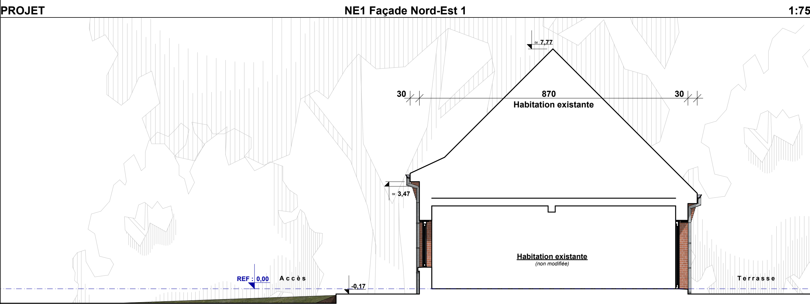
EXISTANT NE1 Façade Nord-Est 1 1:75
