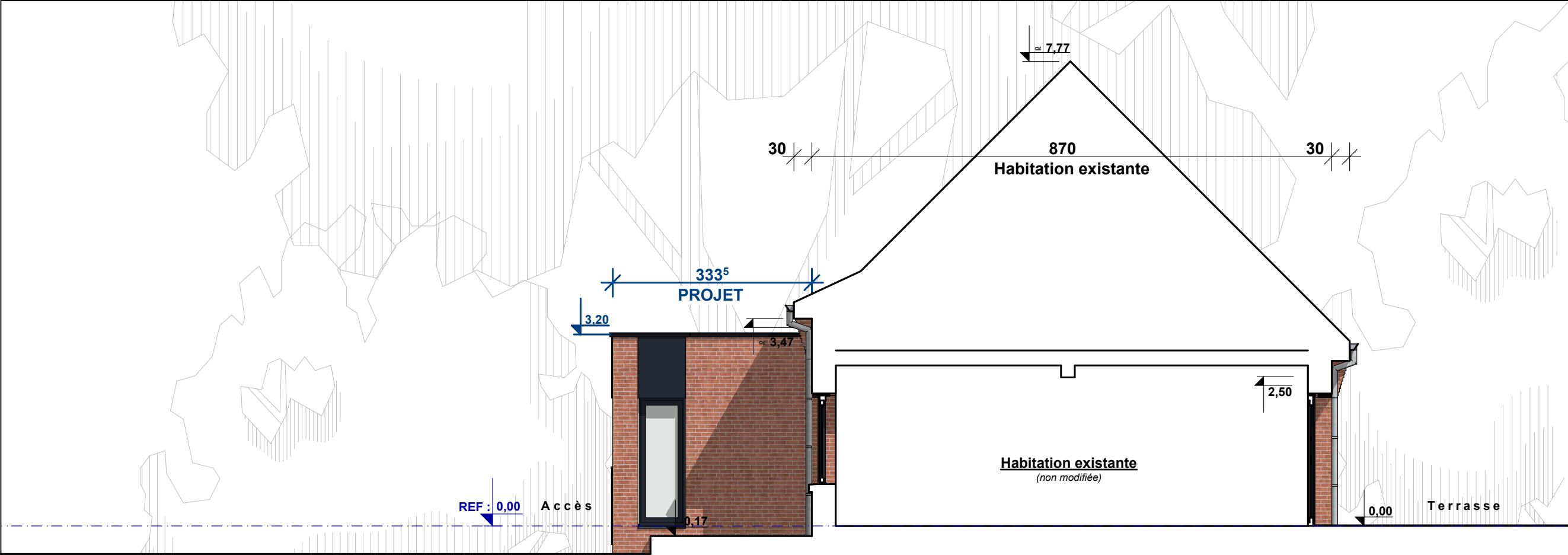
PROJET NE1 Façade Nord-Est 1 1:75
