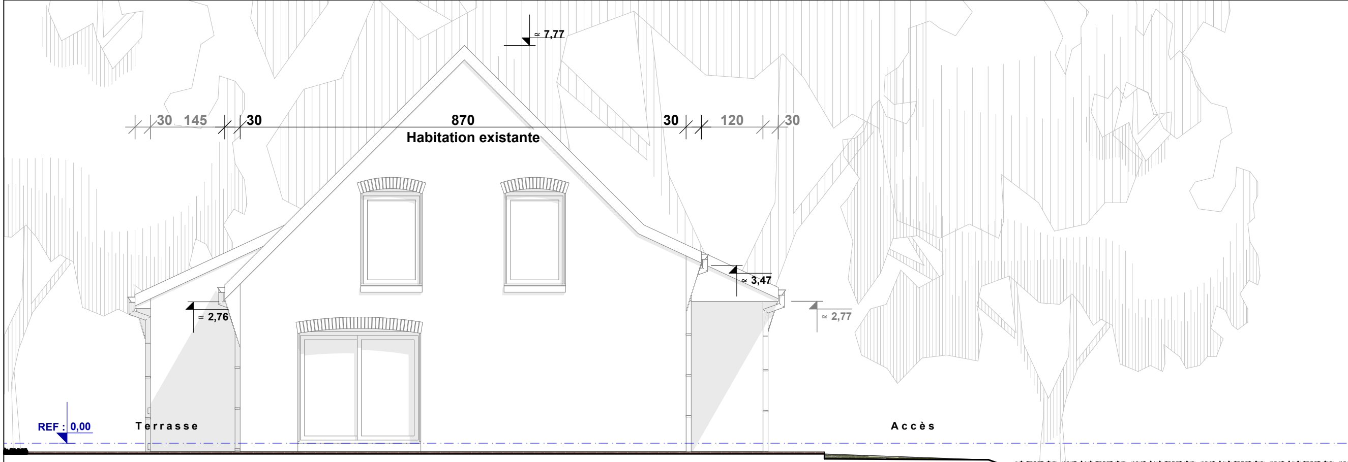
PROJET S01 Façade Sud-Ouest 1 1:75
